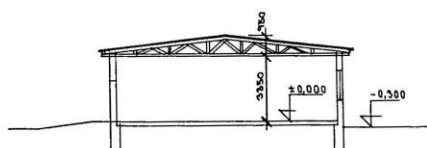
PŘÍČNÝ ŘEZ A-A
